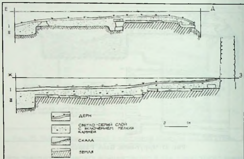
Рис. 32. Чуфут-кале. Баня. Разрезы.
