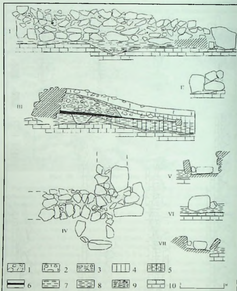
Рис. 28. Постройка №7. Участок раскопа 1983 г. Отдельные детали кладки. I — кладка 12, западный фас; II — кладка 12, южный торец; III — стратиграфический разрез через кладку 12 по линии А-А; IV — каменный ящик, план; V-VII — каменный ящик, внутренняя фасировка стенок (V — северная стенка, VI — западная стенка, VII — южная стенка). 1 — каменный завал; 2 — задержанная часть завала; 3 — каменный завал с суглинистым грунтом; 4 — темновато-серый гумусированный слой; 5 — коричневатого-серый гумусированный суглинок; 6 — углисто-золевая прослойка пожара; 7 — зола; 8 — светлый желтовато-серый суглинок; 9 — элювиальный горизонт из плиток шелушения; 10 — скальное основание плато (известняк).
