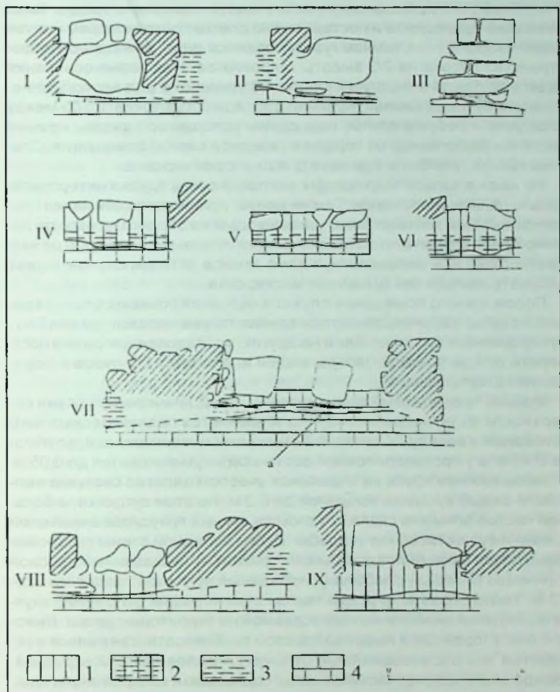
Рис. 17. Постройка №4. Отдельные детали кладки.
