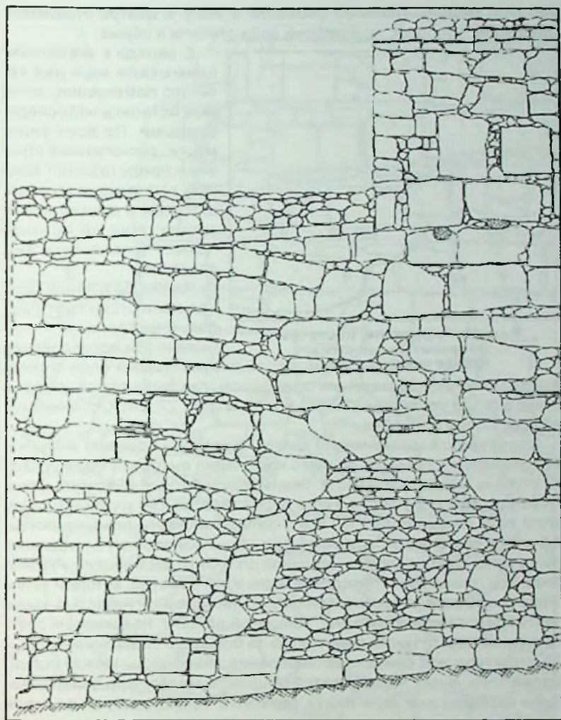
Рис. 22. Чуфут-кале. Восточная оборонительная стена. Южная куртина. Фас участка с внешней стороны.
