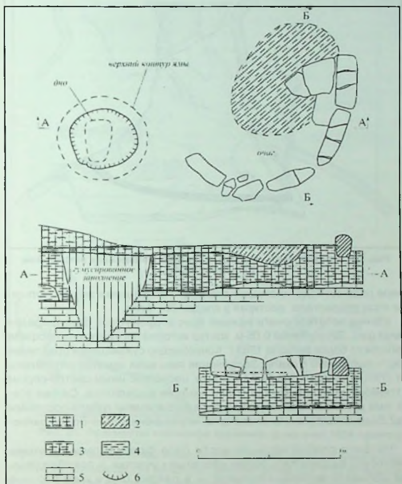
Рис. 29. Постройка №7. Яма и остатки очага. План, разрезы.
