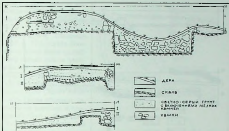
Рис. 31. Чуфут-кале. Баня. Разрезы.
