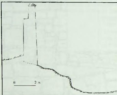
Рис. 23. Чуфут-кале. Восточная оборонительная стена. Южная куртина. Разрез.
