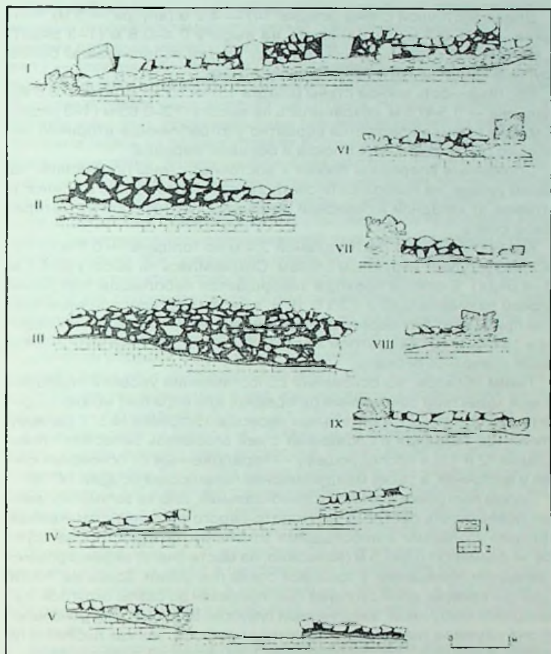
Рис. 8. Постройка №3. Наружная фасировка стен. I — кладка 15, южный фас; II — кладка 14, восточный фас; III — кладка 13, северный фас; IV — кладки 20, 18, южный фас; V — кладки 18, 20, северный фас; VI — кладка 17, восточный фас; VII — кладка 17, западный фас; VIII — кладка 19, восточный фас; IX — кладка 19, западный фас. 1 — светлый желтовато-серый суглинок; 2 — скальное основание плато (известняк).
