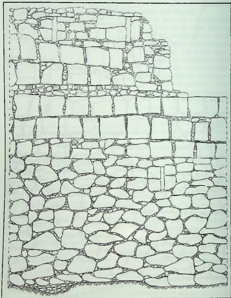
Рис. 25. Чуфут-кале. Восточная оборонительная стена. Северная куртина Фас участка с внешней стороны.
