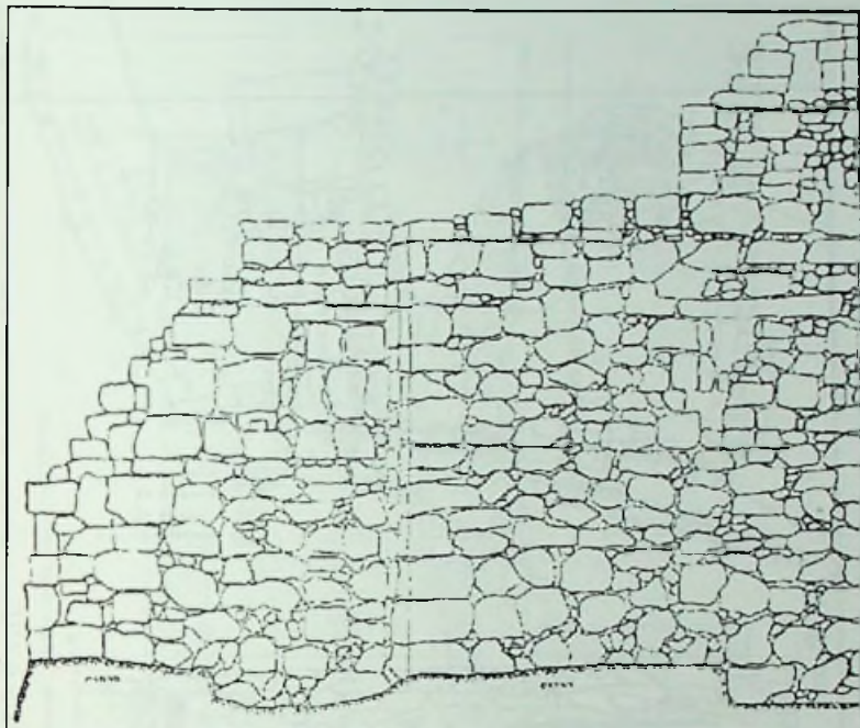
Рис. 26. Чуфут-Кале. Восточная оборонительная стена. Фас на участке раскопа.
