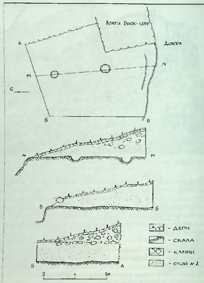
Рис. 14. Чуфут-Кале. Раскоп к северу от ворот Бюк-Капу. План. Разрезы.
