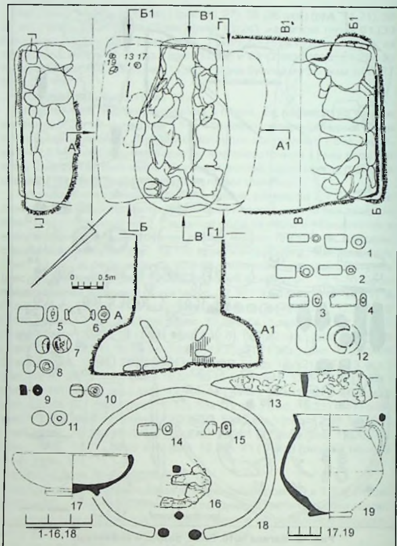
Рис. 13 Могила №11. План, разрезы и инвентарь. Западный подбой: 1-12 — бусы; 16 — фрагмент пряжки; 18 — браслет. Восточный подбой: 13 — нож; 14, 15 — бусы; 17 — красная лаковая миска; 19 — красная лаковая чаша (1-6, 8, 10, 11, 14, 15 — стекло; 7 — сердолик; 9 — гагат; 12, 18 — бронза; 13, 16 — железо).
